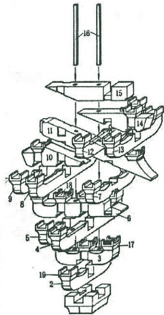
a 分件拼搭示意
